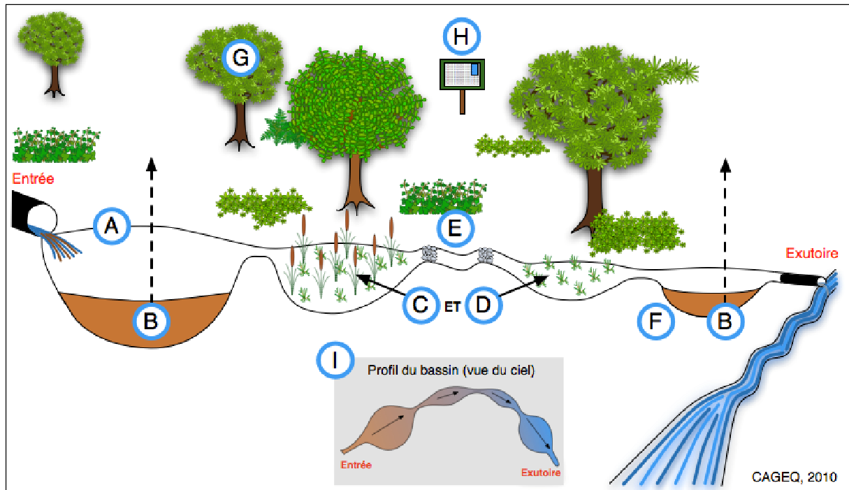
Figure 5. Schéma d'un bassin de rétention et de purification d'eaux pluviales
